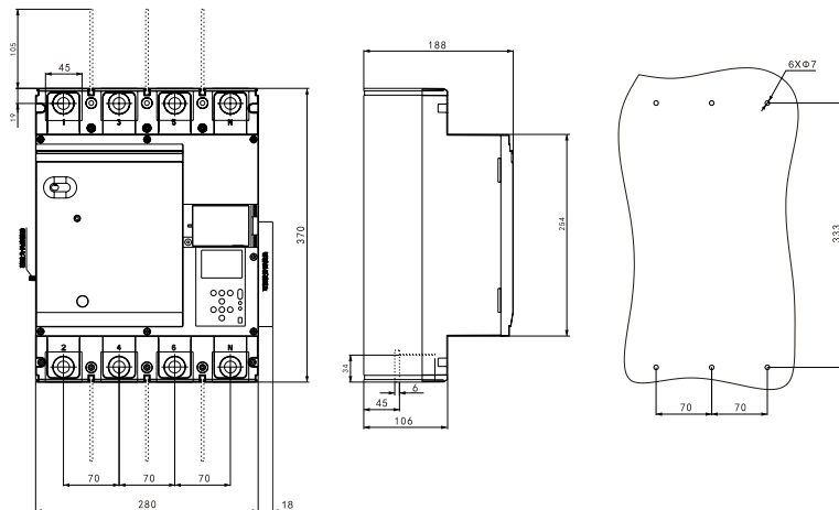
630壳架标准型
