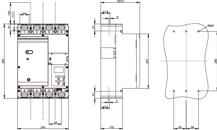
630壳架标准型
